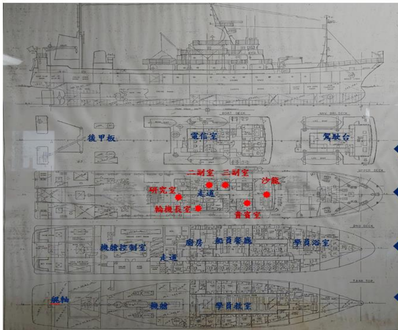
漁訓貳號訓練船隔離配置圖
